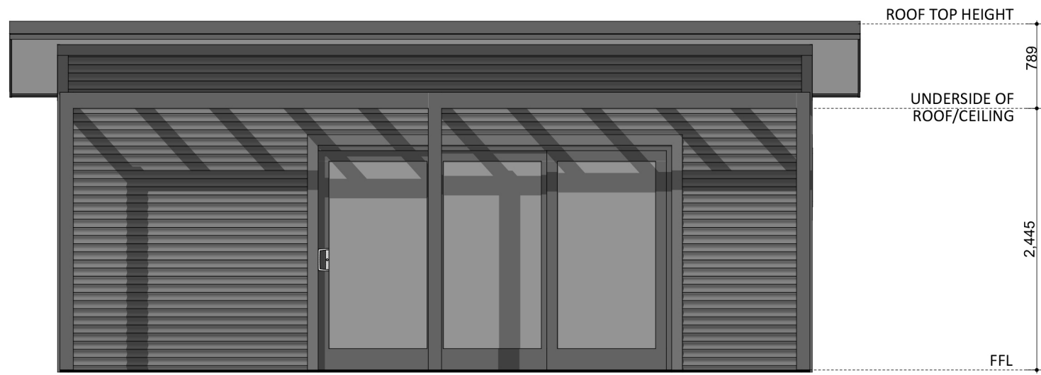
ELEVATION 01
