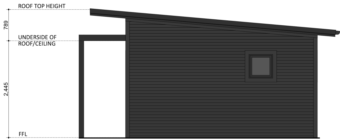
ELEVATION 02
