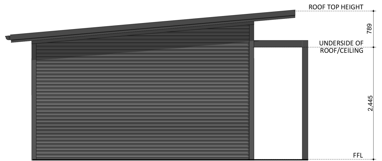
ELEVATION 04
