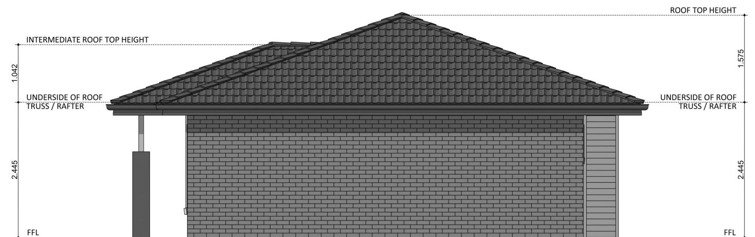
ELEVATION 04
