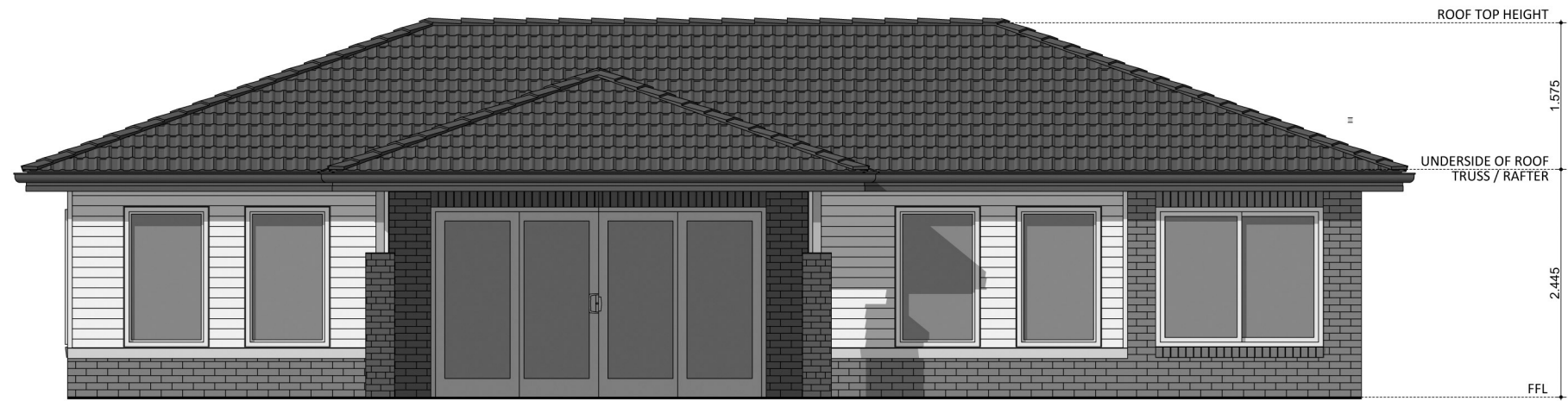
ELEVATION 01
