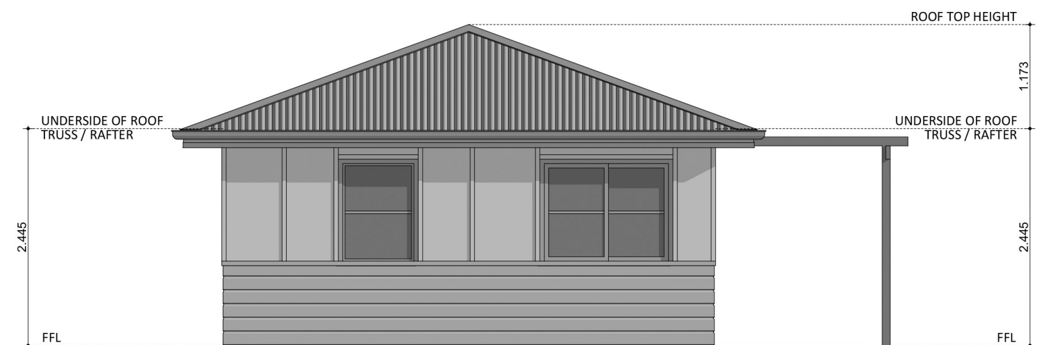
ELEVATION 04
