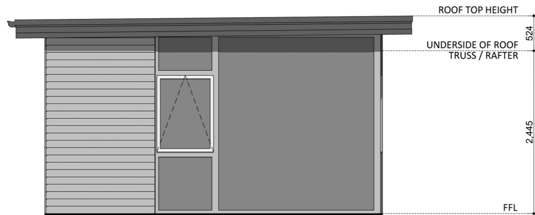
ELEVATION 02
