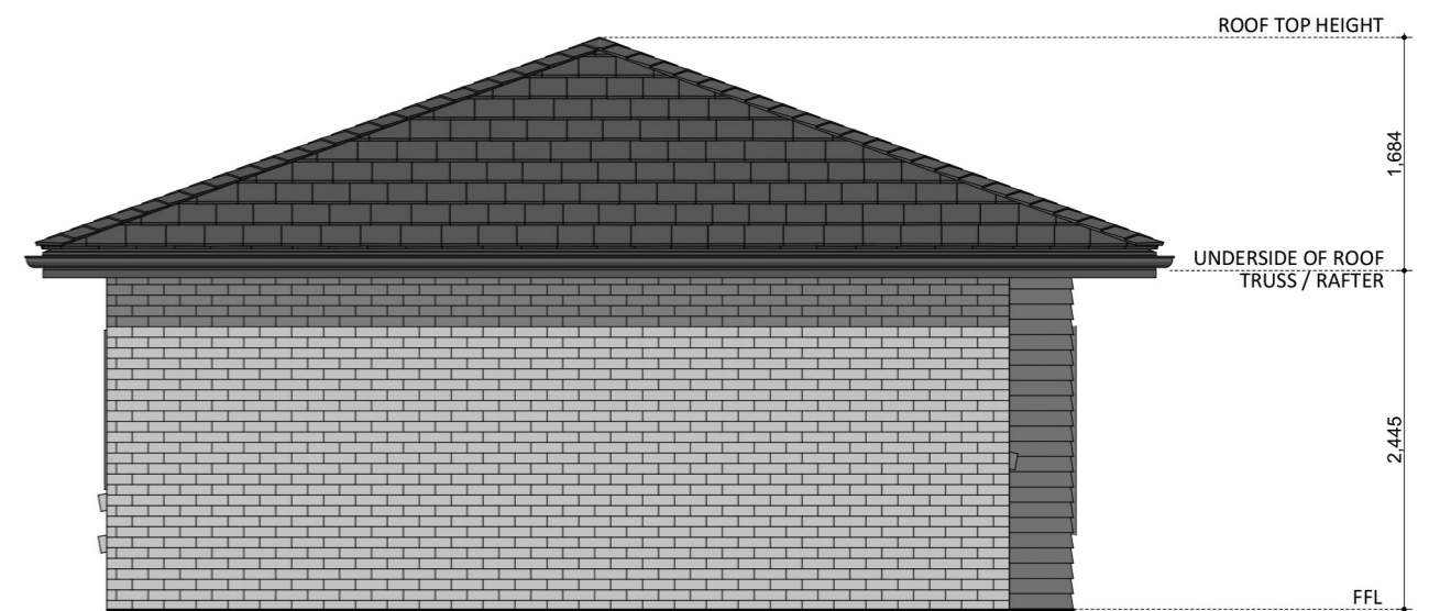
ELEVATION 04
