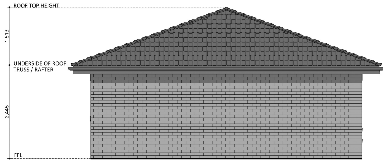
ELEVATION 02
