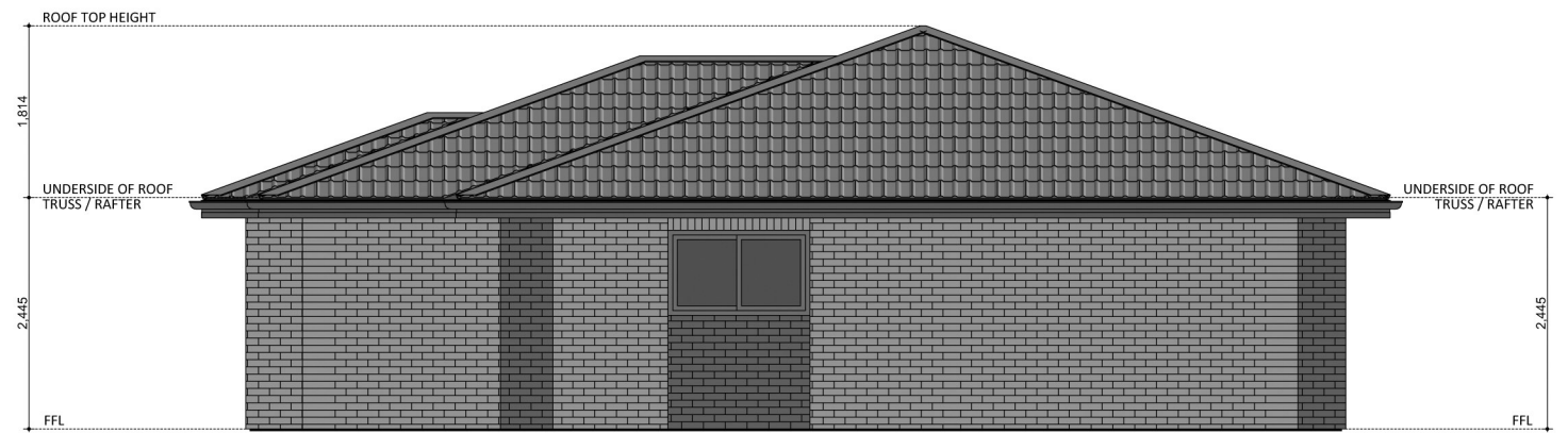
ELEVATION 04
