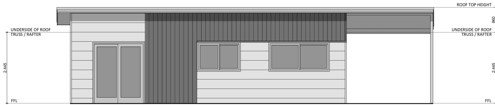
ELEVATION 01
