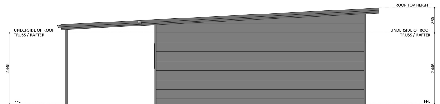
ELEVATION 04
