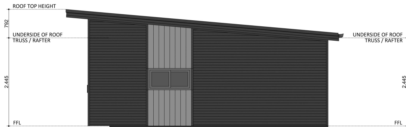
ELEVATION 02
