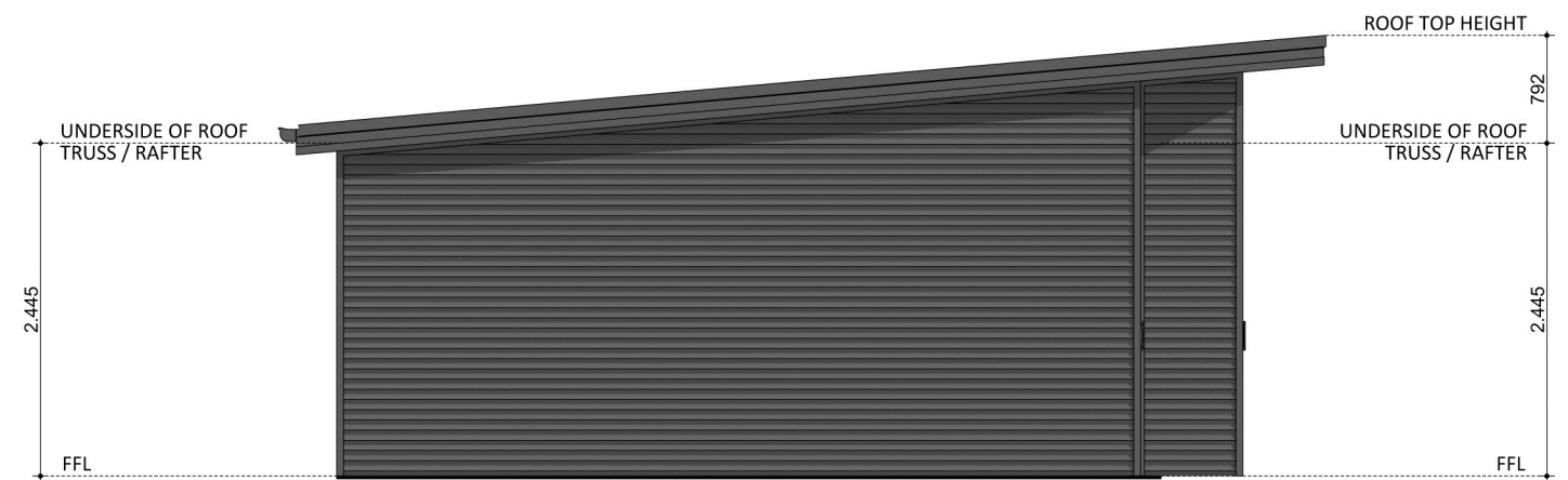
ELEVATION 04
