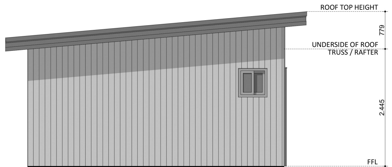
ELEVATION 04
