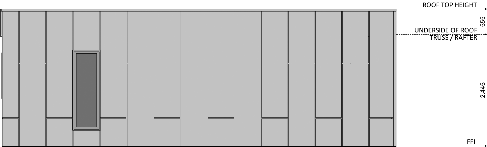
ELEVATION 02
