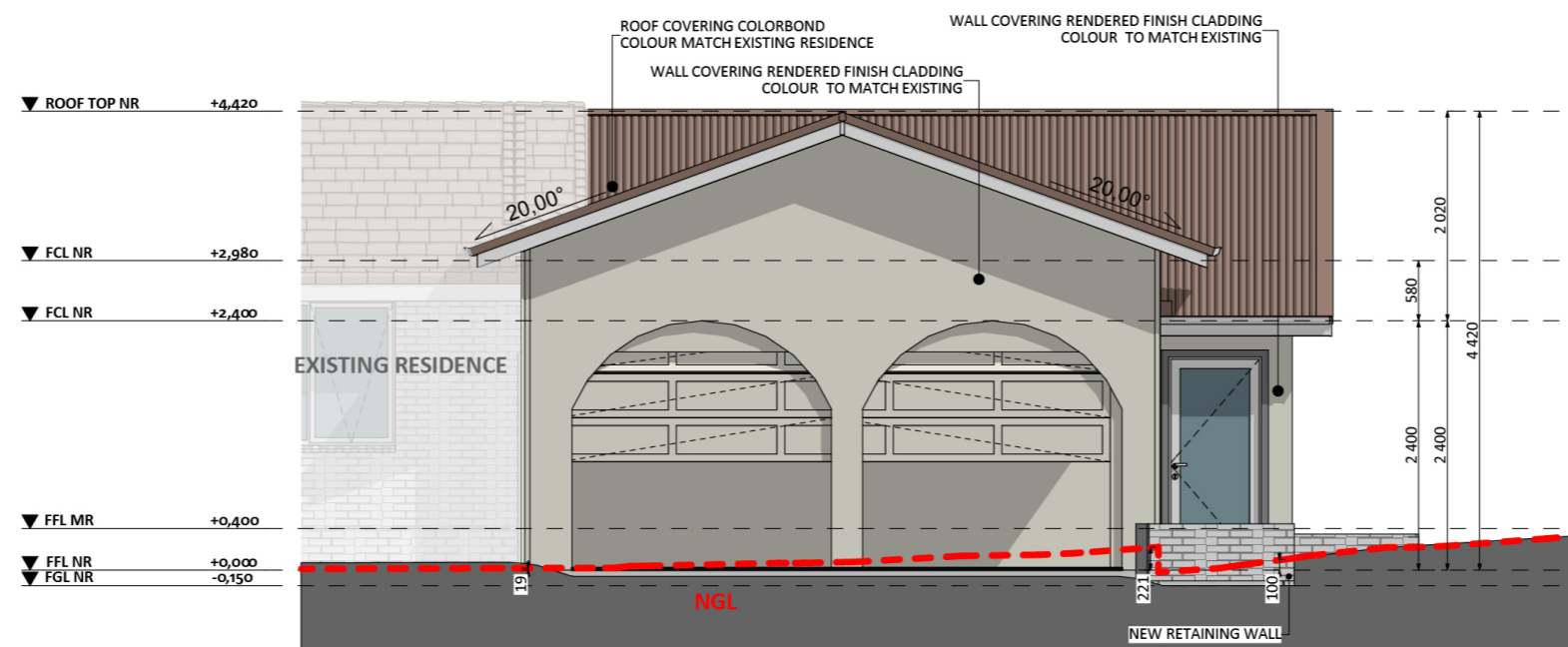
ELEVATION 02
