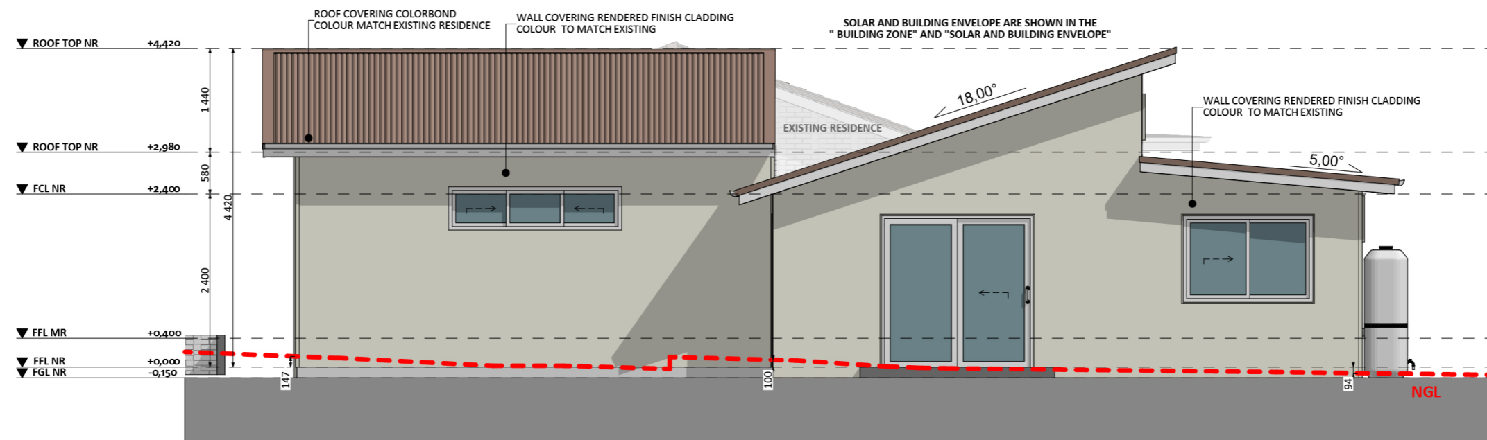
ELEVATION 01
