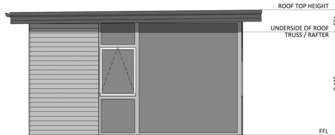
ELEVATION 02
