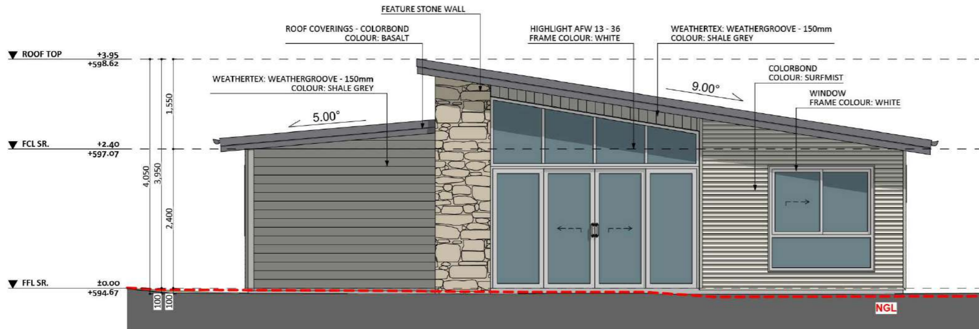
ELEVATION 01
