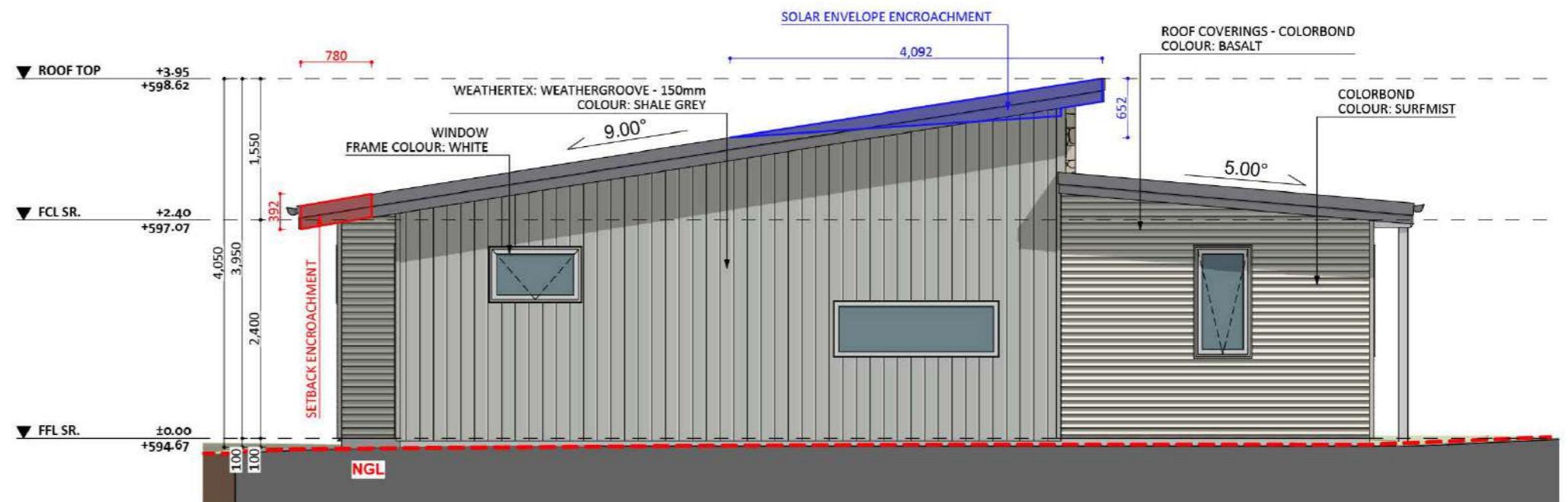
ELEVATION 04
