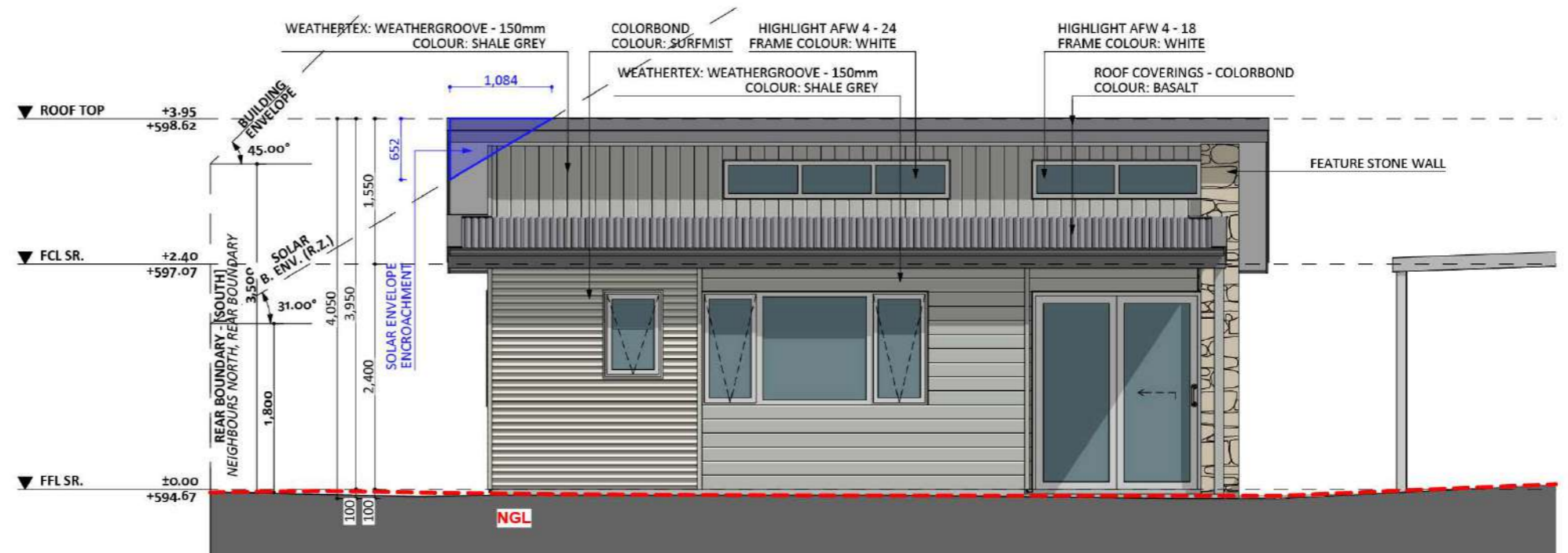
ELEVATION 02
