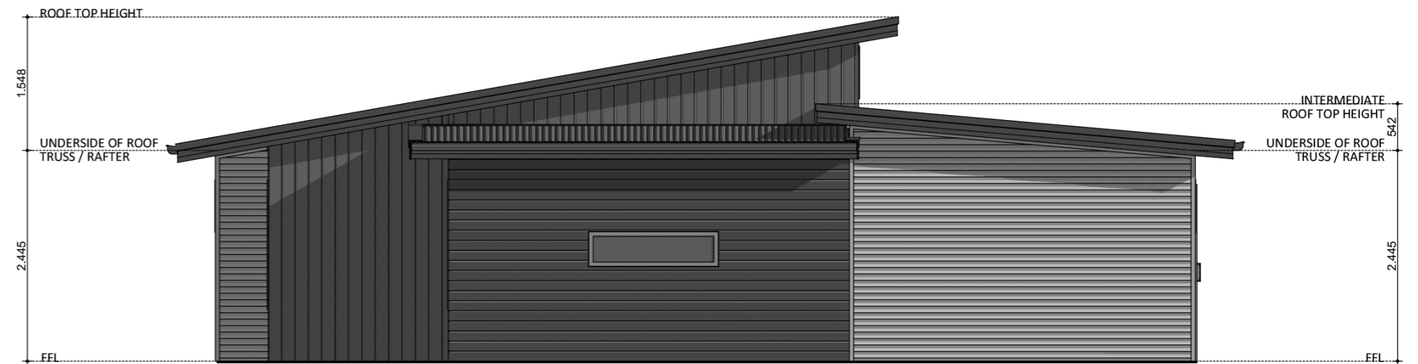
ELEVATION 04
