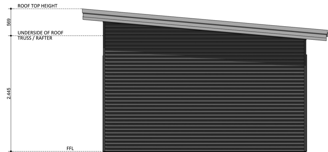
ELEVATION 02
