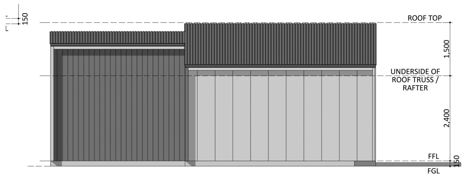
ELEVATION 4
