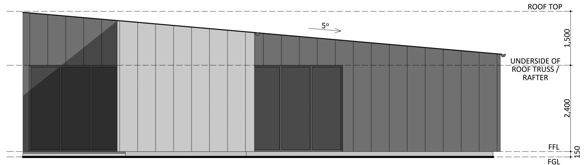
ELEVATION 2
