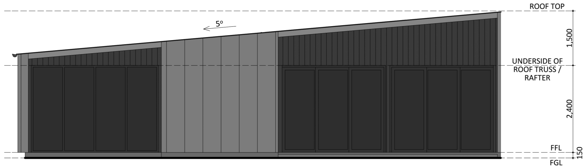
ELEVATION 3
