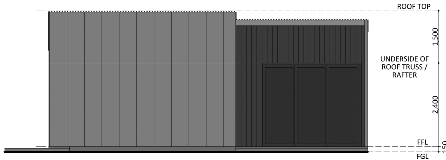
ELEVATION 1
