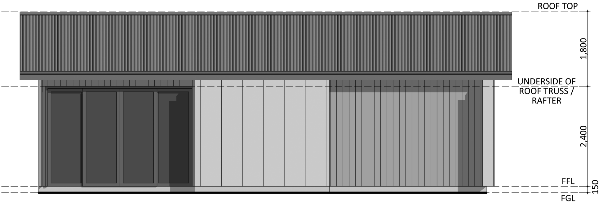
ELEVATION 2
