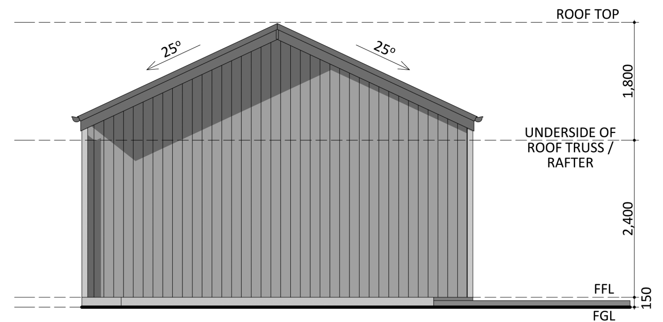
ELEVATION 4
