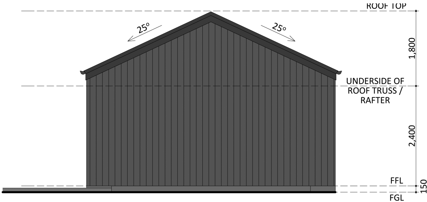
ELEVATION 1
