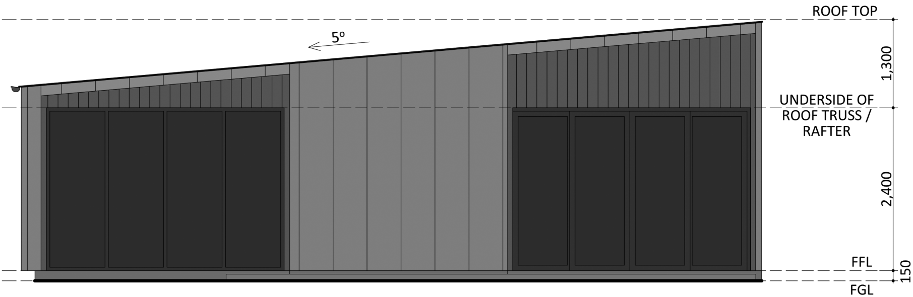
ELEVATION 3
