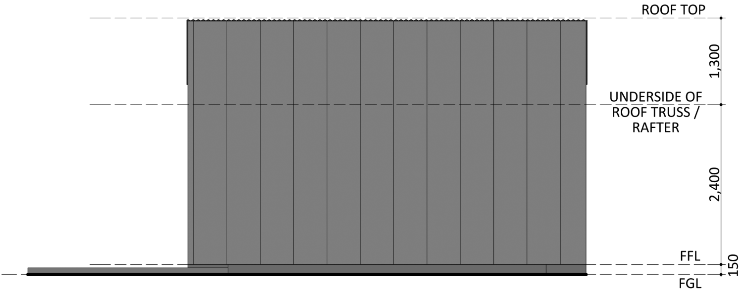
ELEVATION 1
