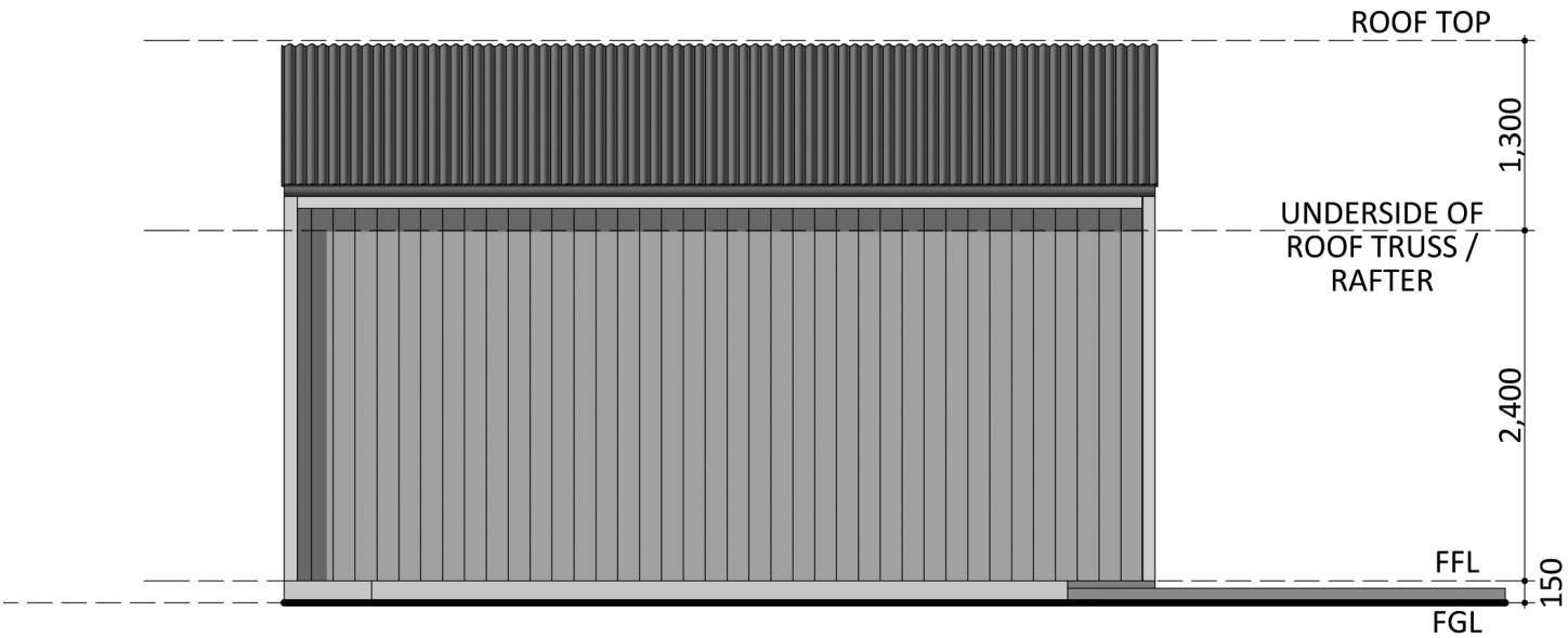
ELEVATION 4
