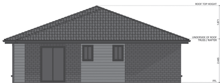
ELEVATION 04
