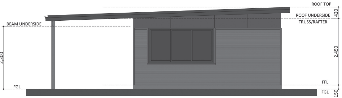
ELEVATION 02
