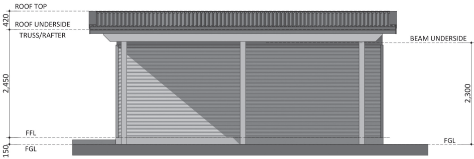
ELEVATION 04
