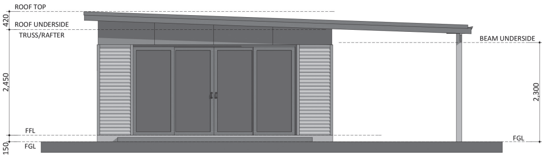
ELEVATION 01
