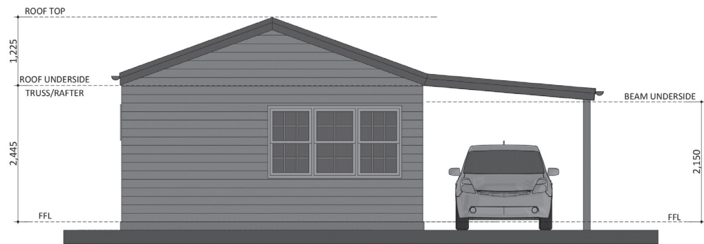
ELEVATION 02
