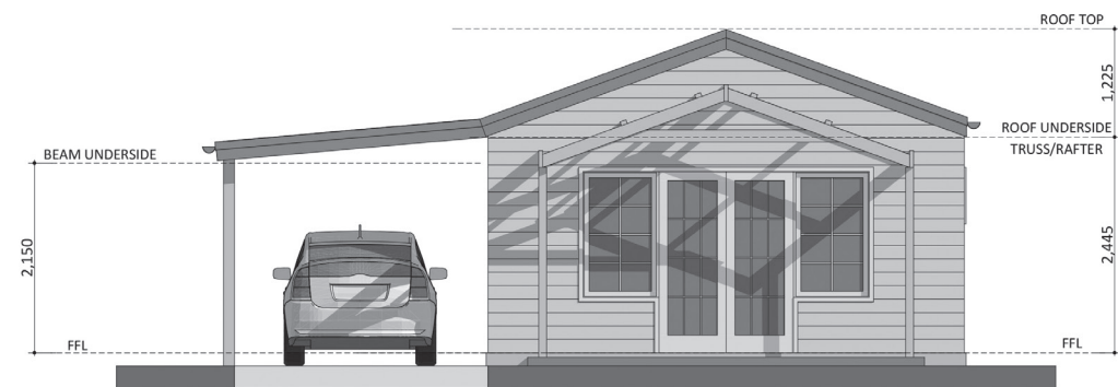
ELEVATION 01
