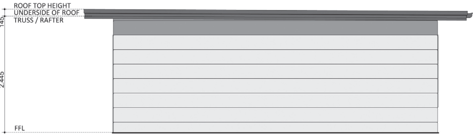
ELEVATION 02
