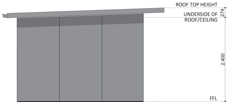
ELEVATION 04
