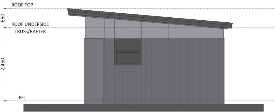
ELEVATION 04
