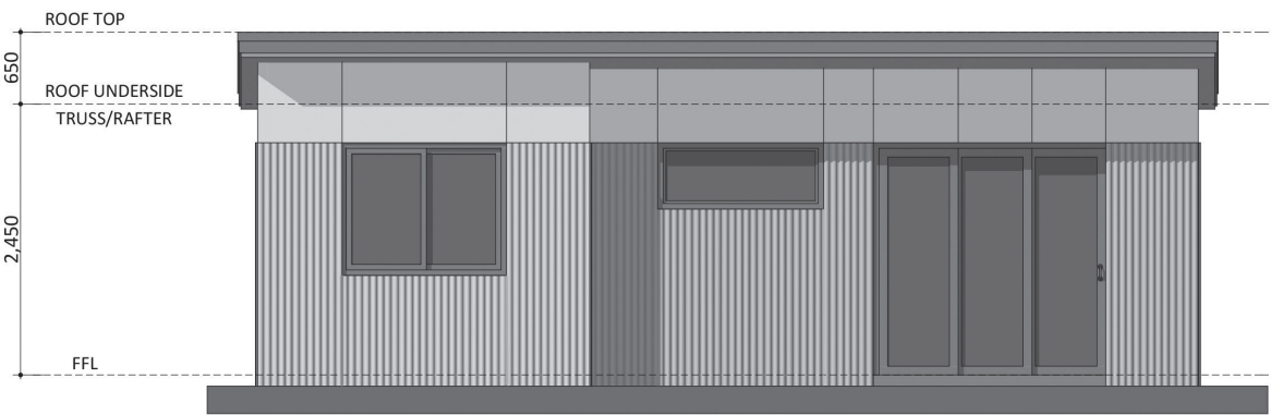
ELEVATION 02
