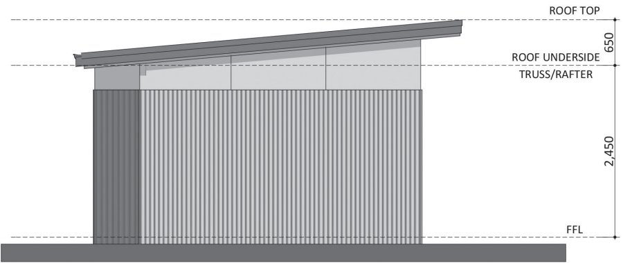
ELEVATION 01
