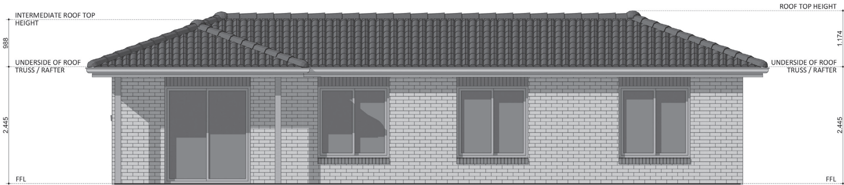
ELEVATION 01
