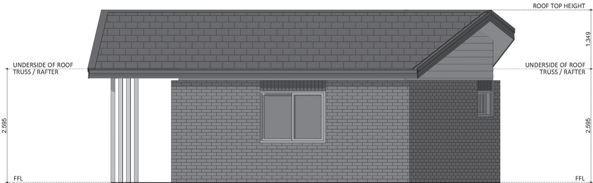
ELEVATION 01
