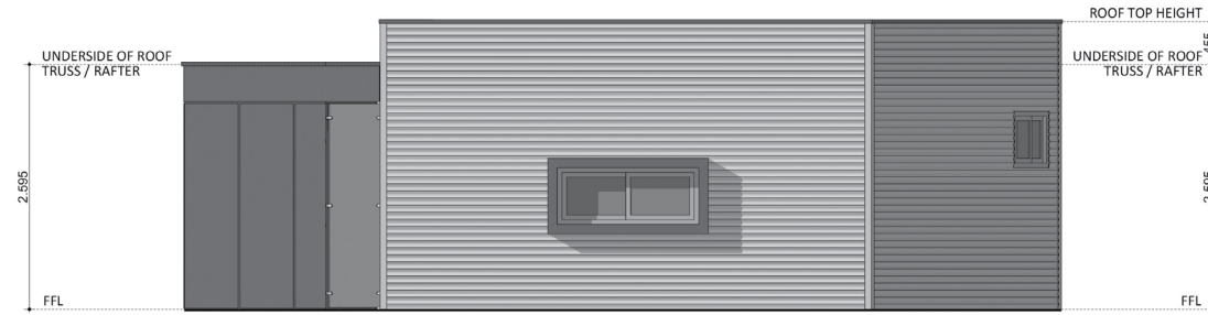
ELEVATION 01
