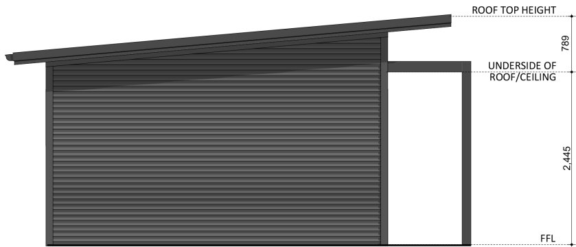
ELEVATION 04
