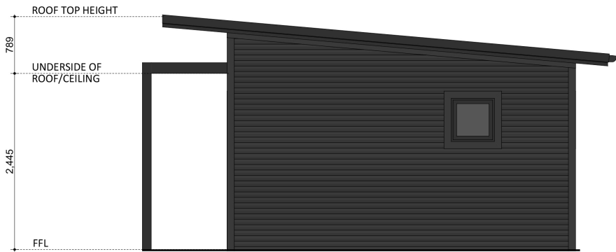
ELEVATION 02
