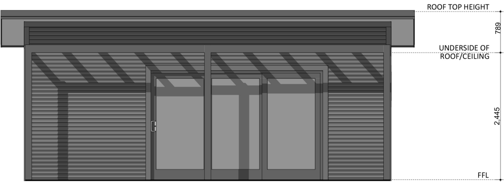
ELEVATION 01
