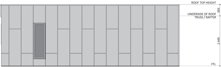
ELEVATION 02
