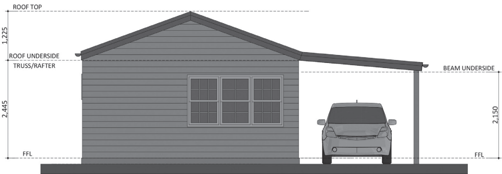
ELEVATION 02
