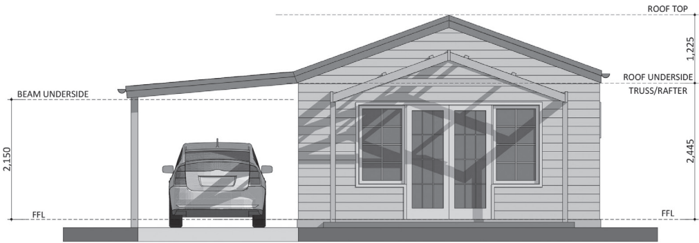
ELEVATION 01
