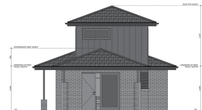
ELEVATION 04
