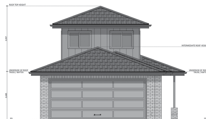
ELEVATION 02
