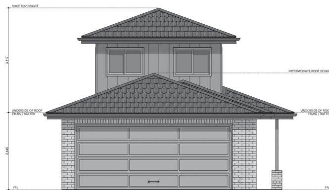
ELEVATION 02
