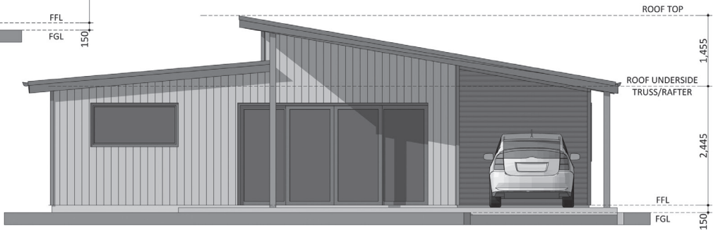
ELEVATION 2
