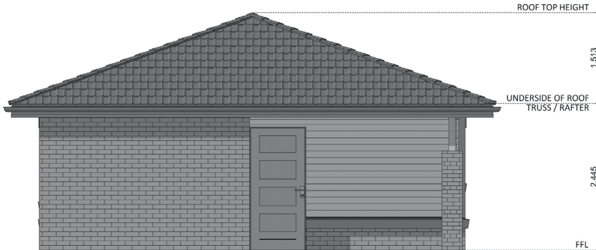
ELEVATION 04
