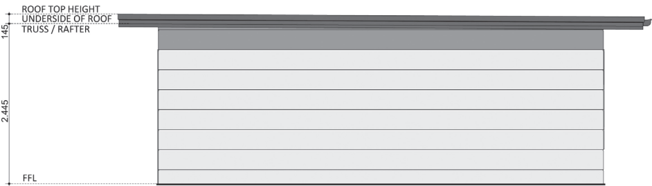
ELEVATION 02
