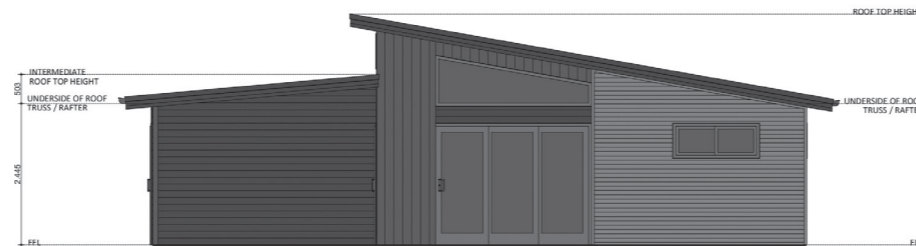
ELEVATION 02
