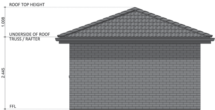
ELEVATION 02
