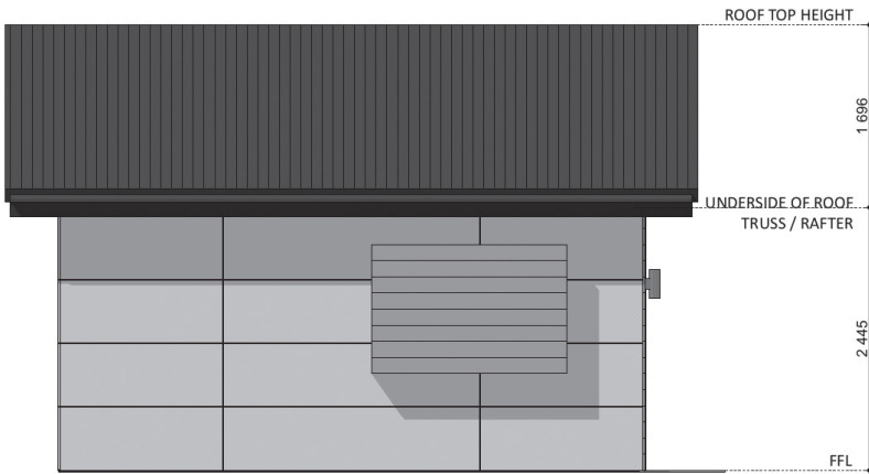
ELEVATION 04
