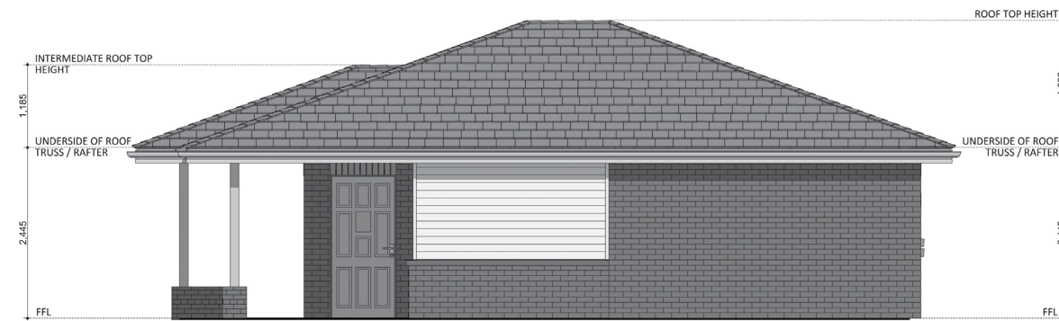
ELEVATION 02
