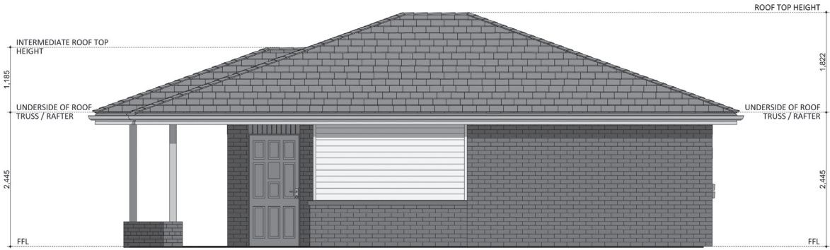
ELEVATION 02
