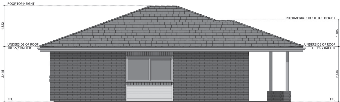
ELEVATION 04
