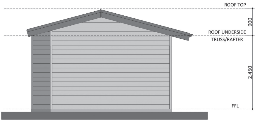
ELEVATION 01
