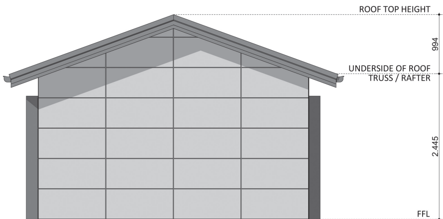
ELEVATION 04
