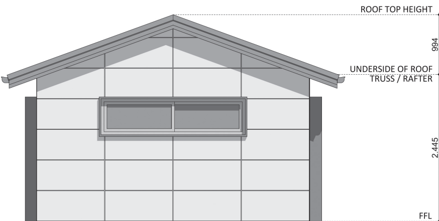
ELEVATION 02
