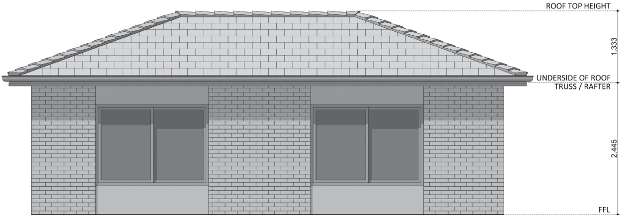
ELEVATION 01
