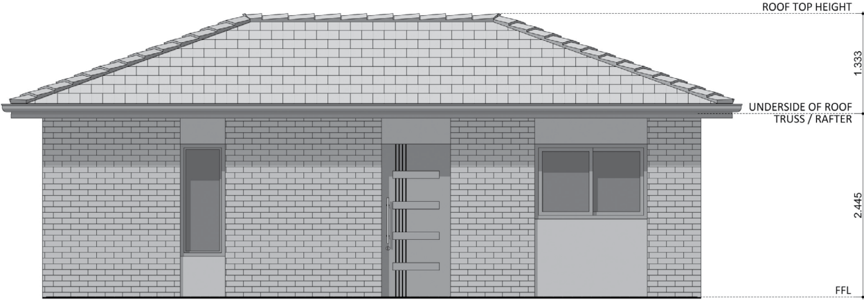
ELEVATION 01
