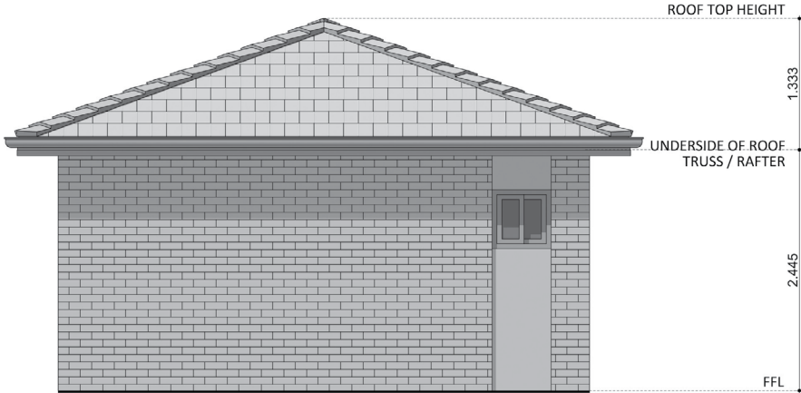
ELEVATION 04
