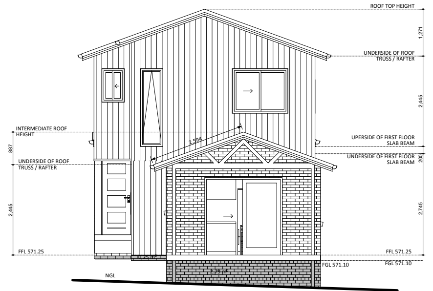
ELEVATION 04
