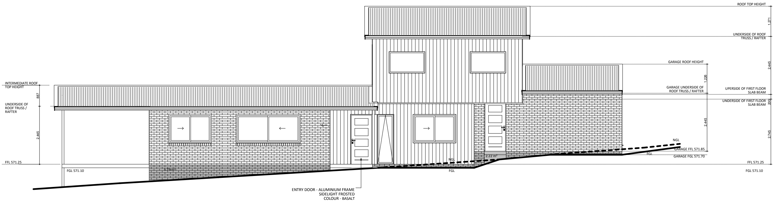
ELEVATION 01
