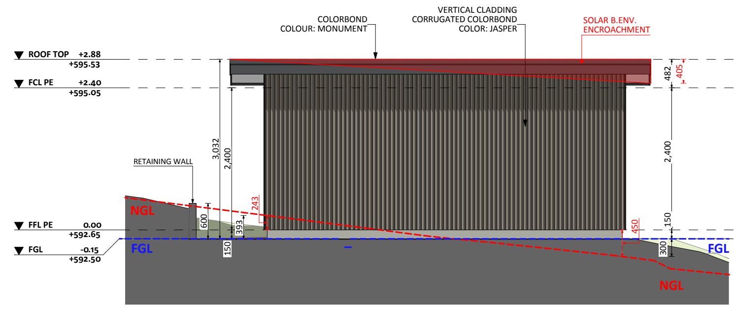
ELEVATION 04
