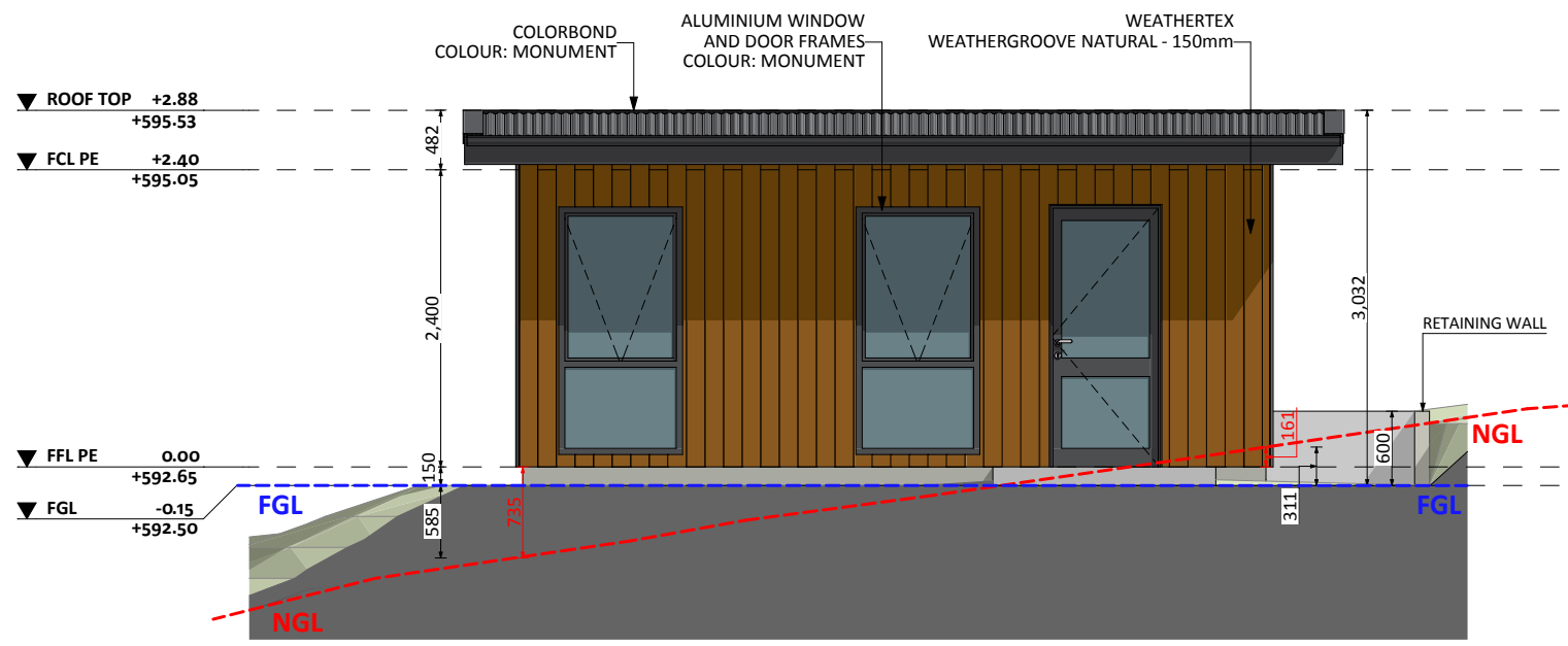
ELEVATION 01
