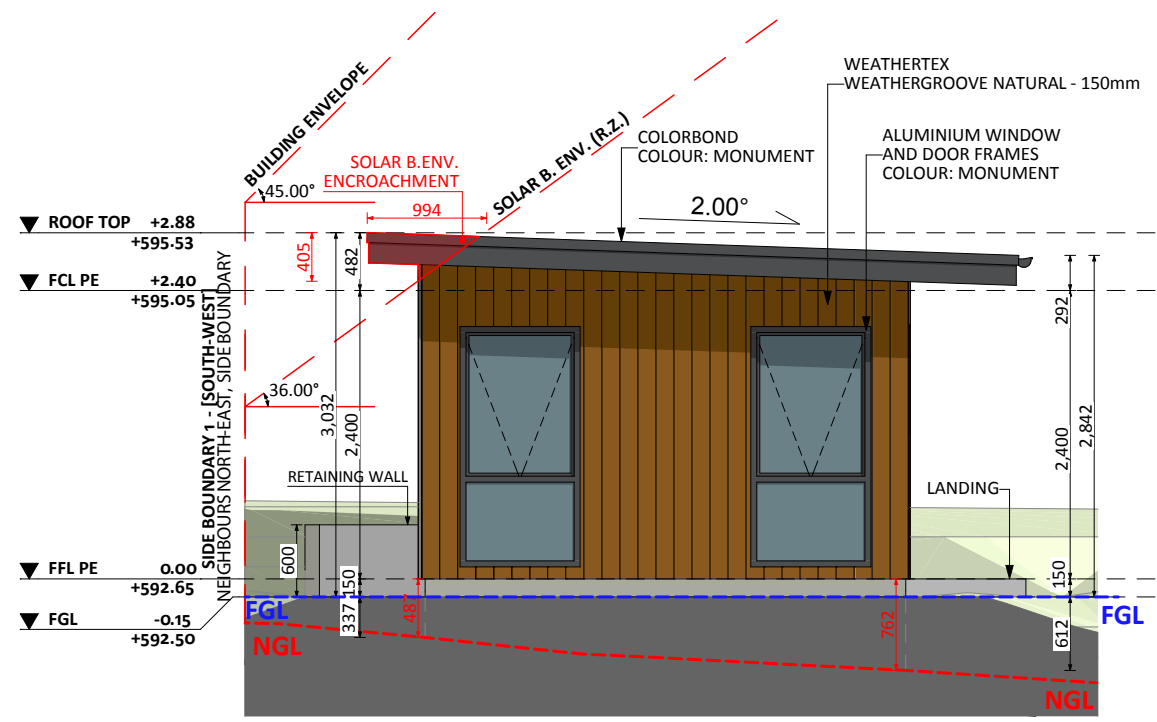
ELEVATION 02
