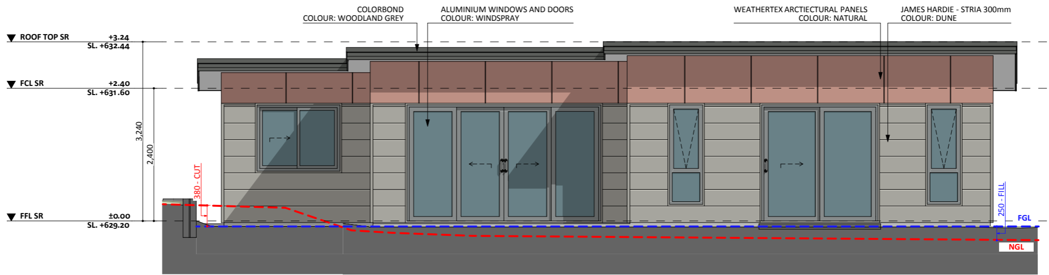
ELEVATION 01
