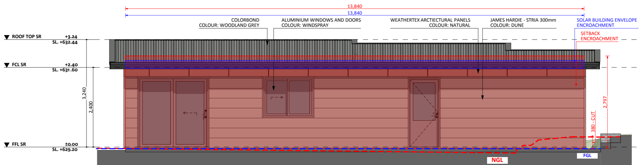
ELEVATION 04
