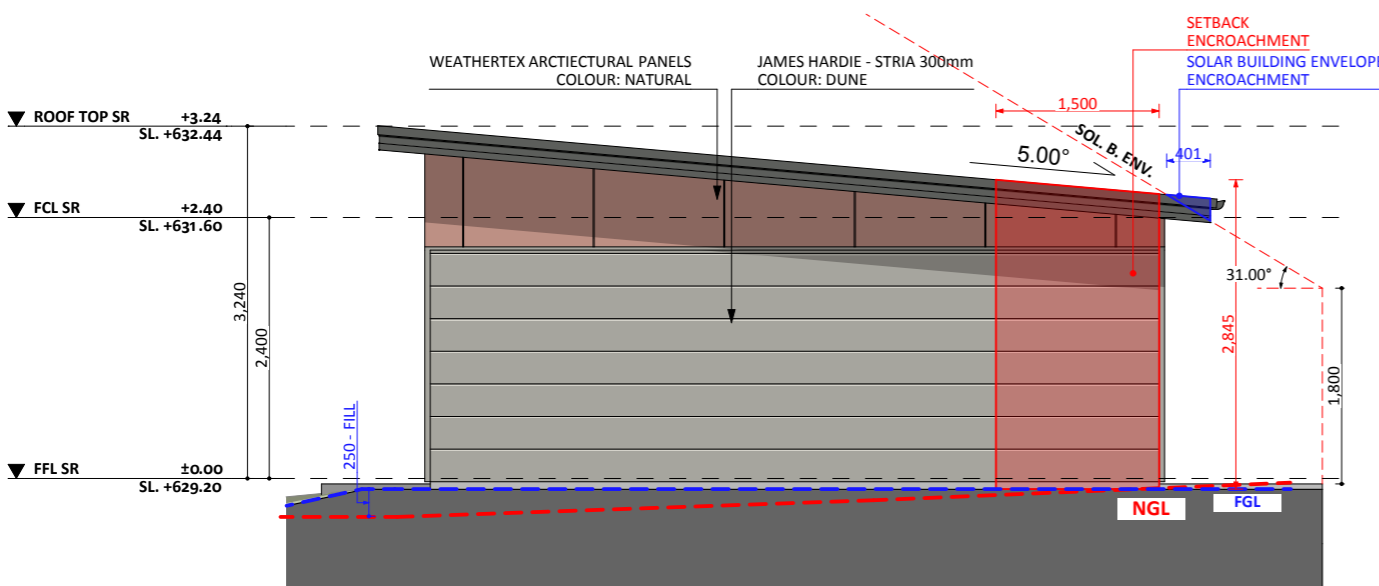
ELEVATION 02
