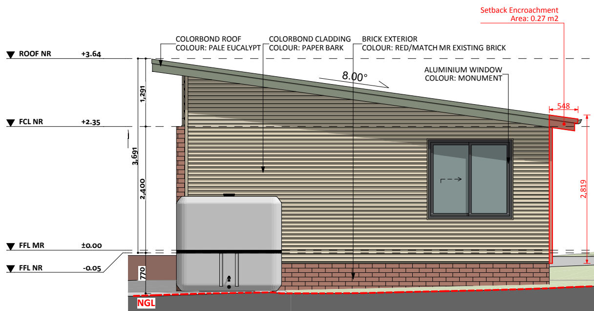
ELEVATION 02
