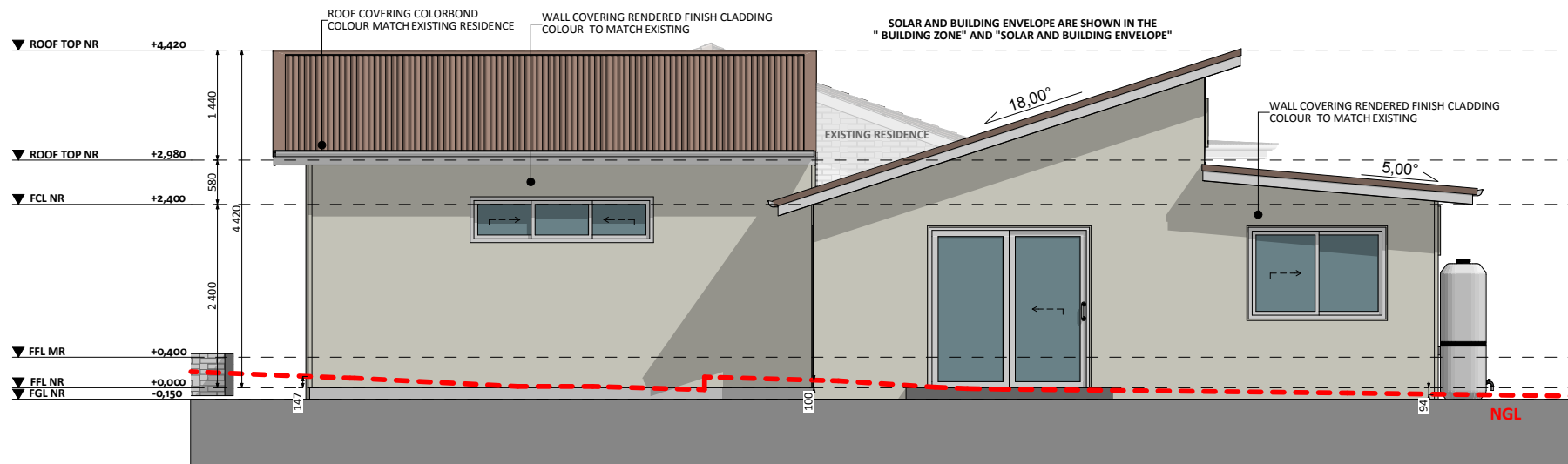
ELEVATION 01
