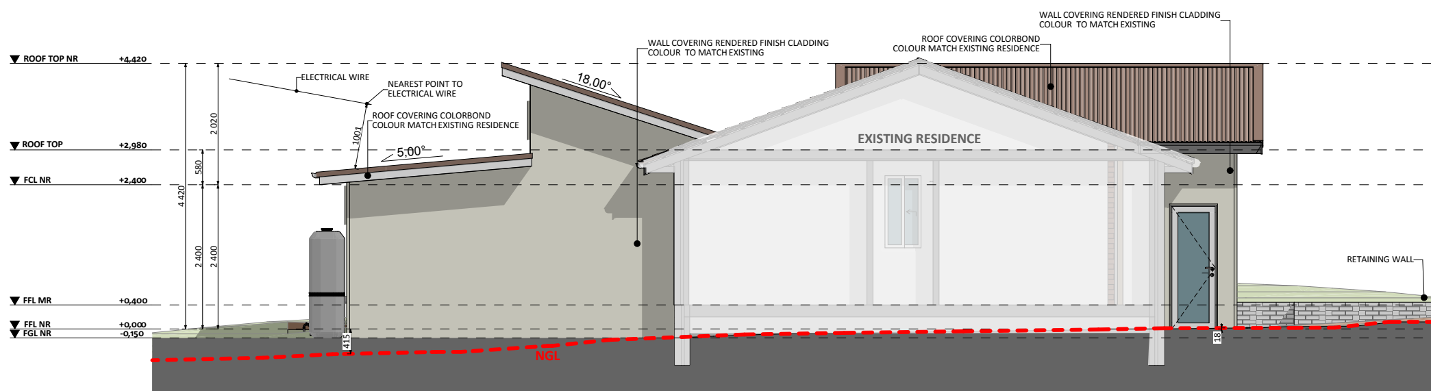
ELEVATION 04
