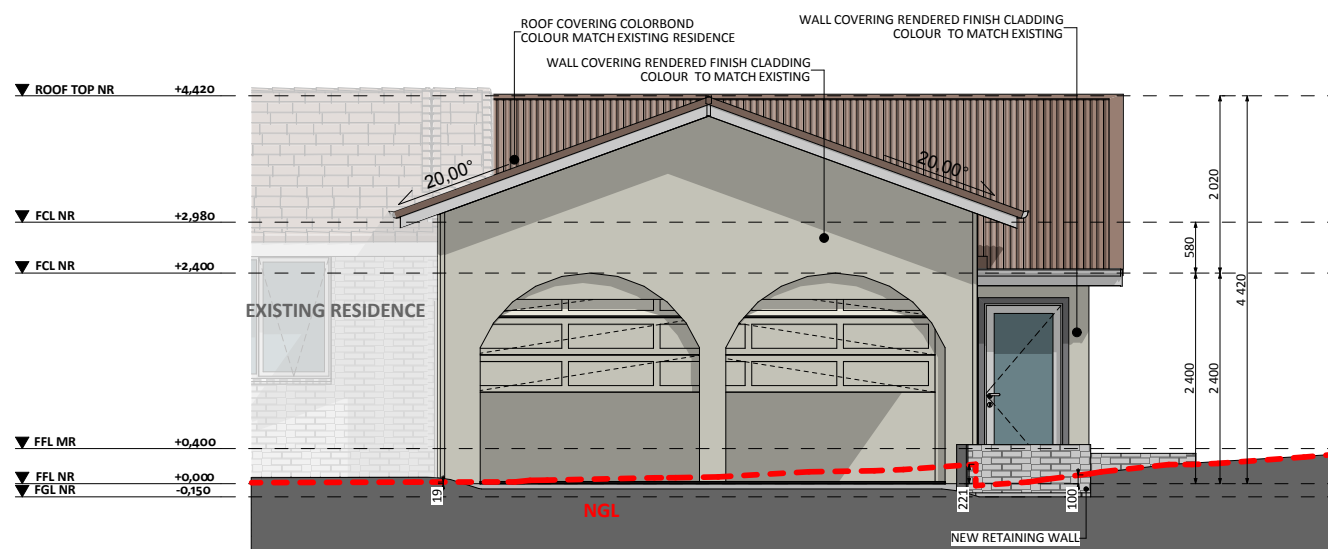
ELEVATION 02
