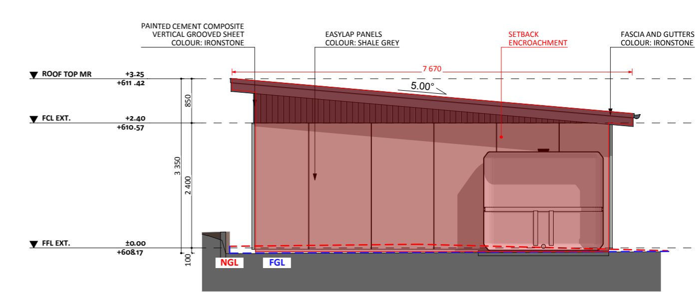
ELEVATION 04
