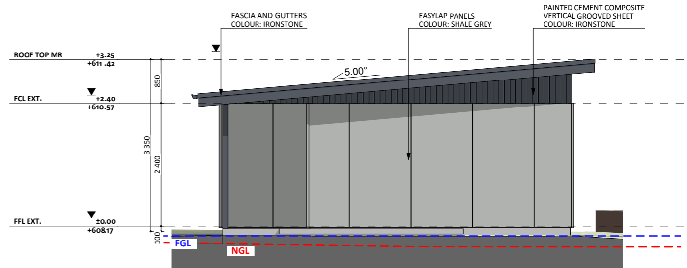
ELEVATION 02
